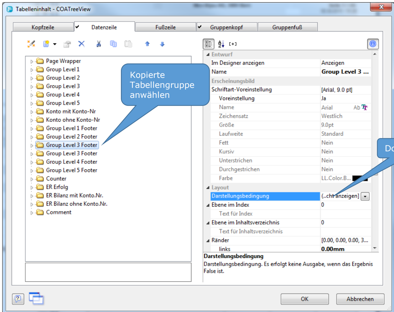
Abbildung 8: Kopierter Tabelleninhalt Darstellungsbedingung
