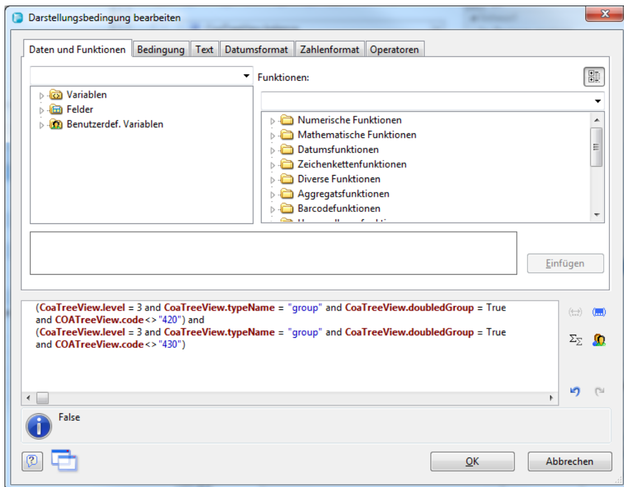
Abbildung 11: Formel um Darstellungsbedingung auszuschliessen
